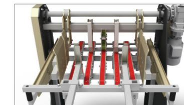
吸引ベルト付きの2重搬送システムで幅広い資材を搬送可能です。
